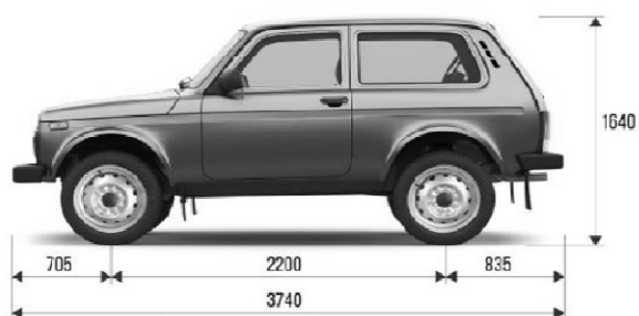
LADA 4X4 CLASSIC
